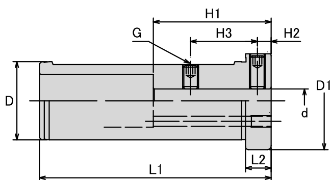
TSB40 専用スリーブ Coolant/Size Reduction Sleeve for TSB40
